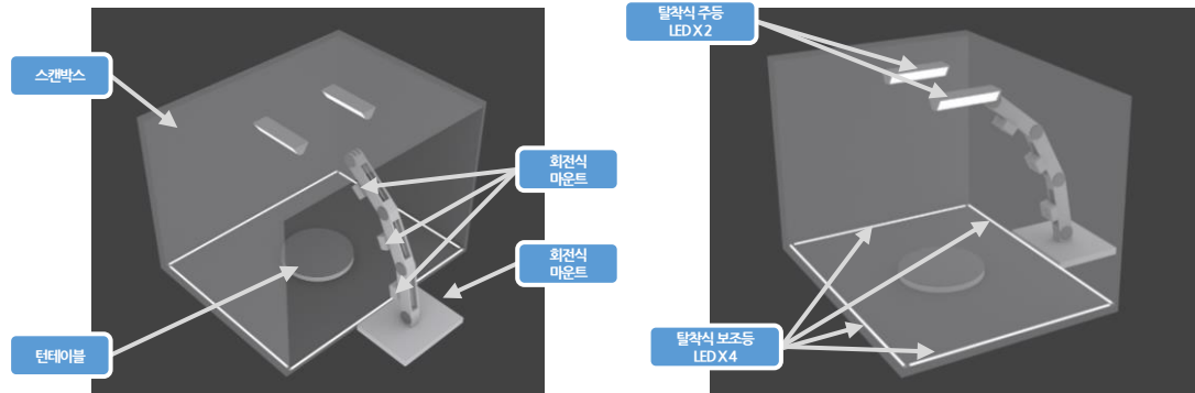
[스캔박스 구성도_하드웨어]
