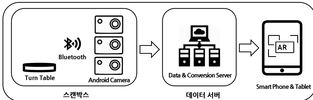
[2D영상 기반 3D 데이터 생성시스템 하드웨어 구조도]
